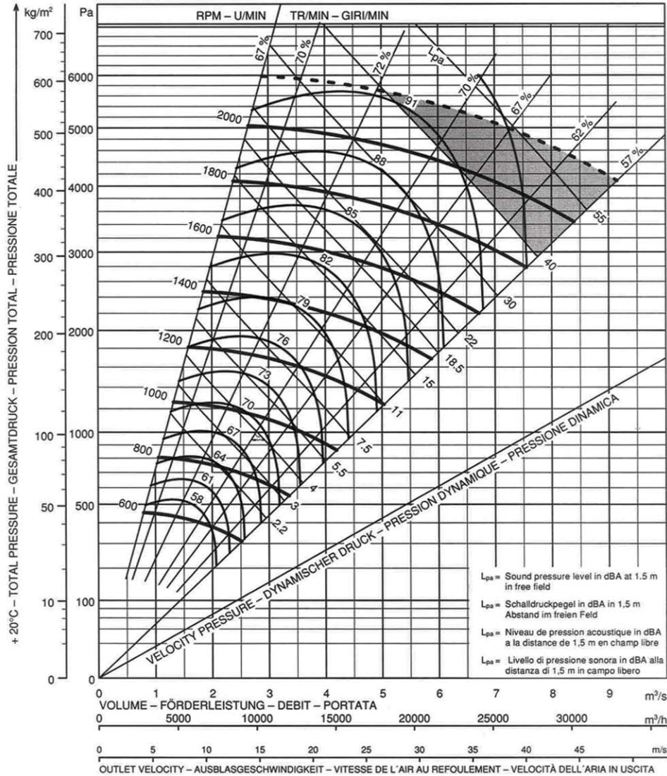
PM 740 Girante \phi 740 Bocca aspirante \phi 550 - Bocca premente 405 x 460
