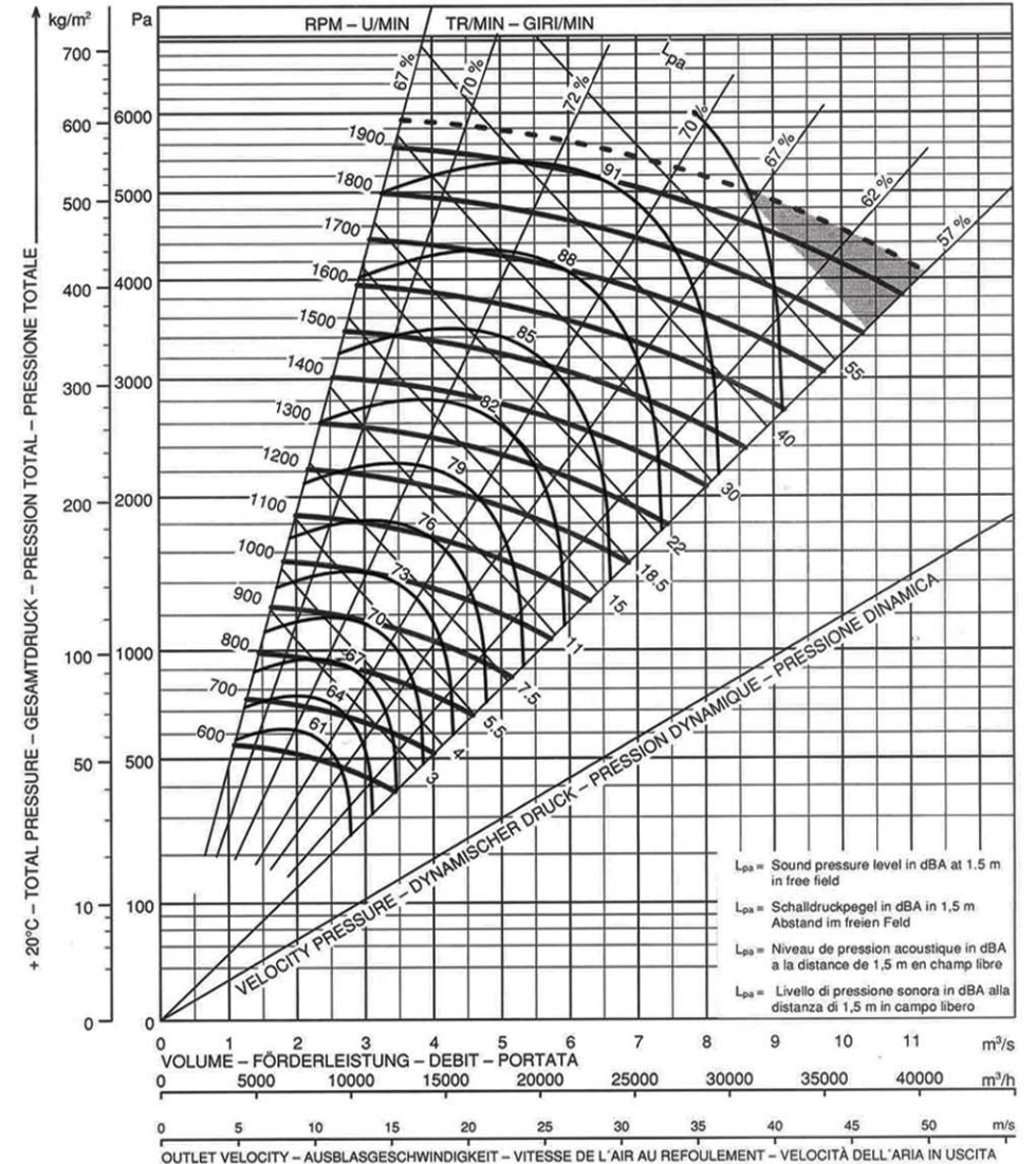
PM 820 Girante \phi 829 Bocca aspirante \phi 600 - Bocca premente 446 x 500
