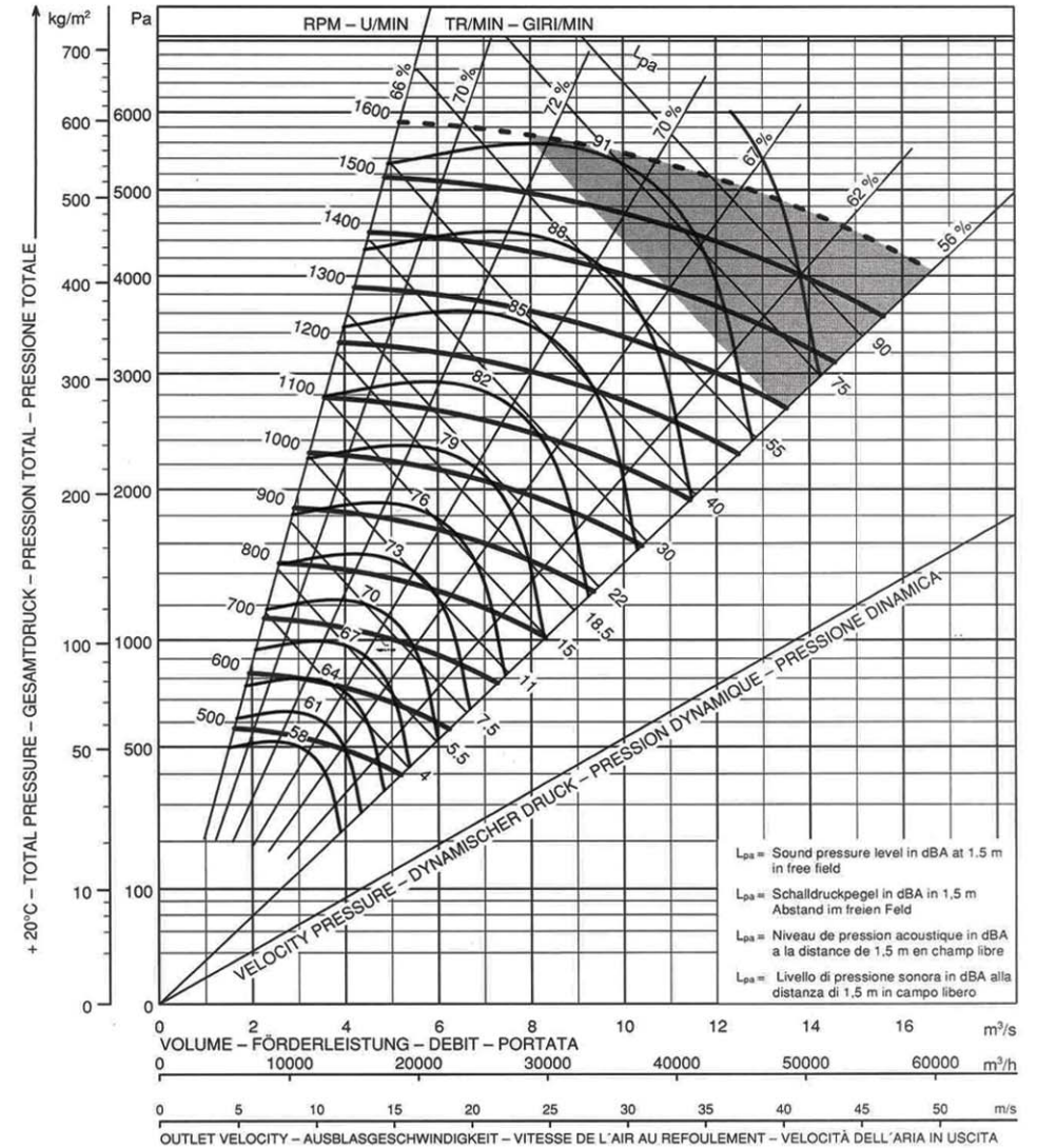
PM 1000 Girante \phi 1000 Bocca aspirante \phi 700 - Bocca premente 540 x 610
