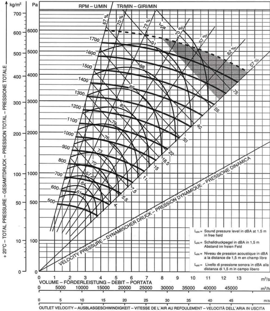
PM 900 Girante \phi 910 Bocca aspirante \phi 650 - Bocca premente 495 x 554
